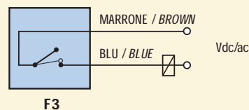
CONTATTO BISTABILE BISTABLE CONTACT
