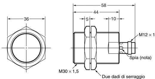
E2A-M30KS15-M1-□□/E2A-S30KS15-M1-□
